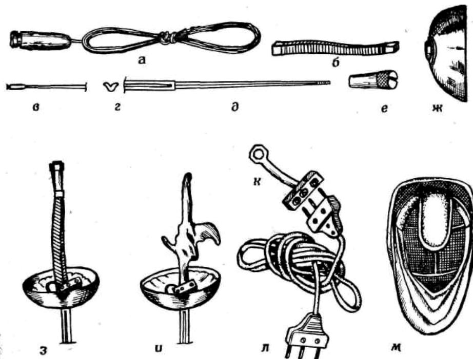
Рис. 151. Электрофицированная шпага, ее составные части и маска:
