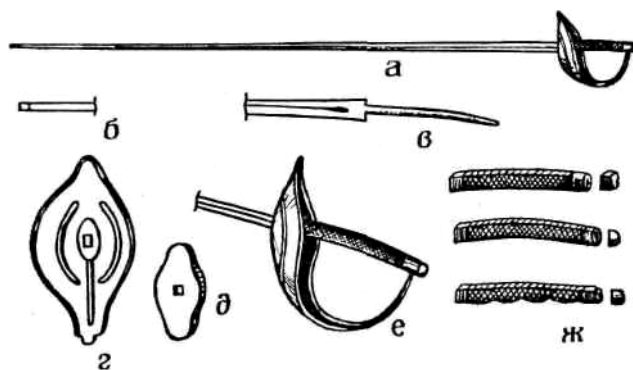
Рис. 127. Спортивная сабля и ее составные части: а — общий вид; б — пуговка острия; в — хвост клинка; г — гарда; д — прокладка; е — вид сбоку; ж — формы рукояток.
