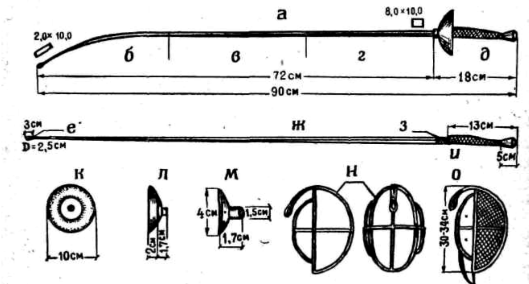
Рис. 48. Рапира из синтетического материала:
