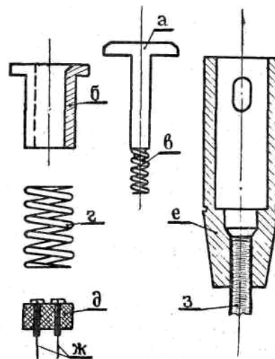
Рис. 153. Наконечник шпаги в разобранном виде:
