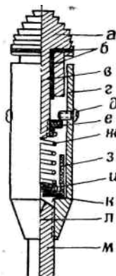
Рис. 50. Наконечник электрофицированной рапиры:
