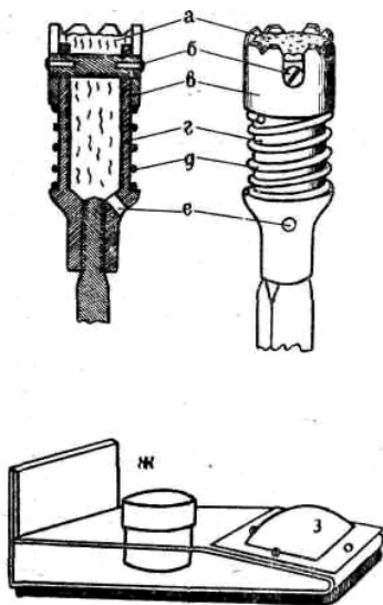
Рис. 49. Красящий наконечник — фиксатор уколов:
