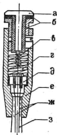
Рис. 152. Общий вид электрофицированного наконечника шпаги.
